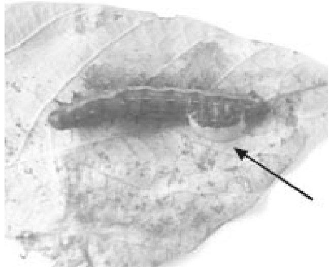
Gambar 1. Bagian integumen larva S. litura yang mudah pecah mengeluarkan polyhedra (Bedjo, 2003).
